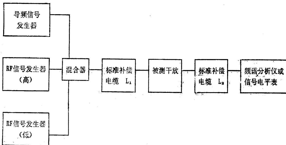
图5 AGC和斜率补偿特性测量
