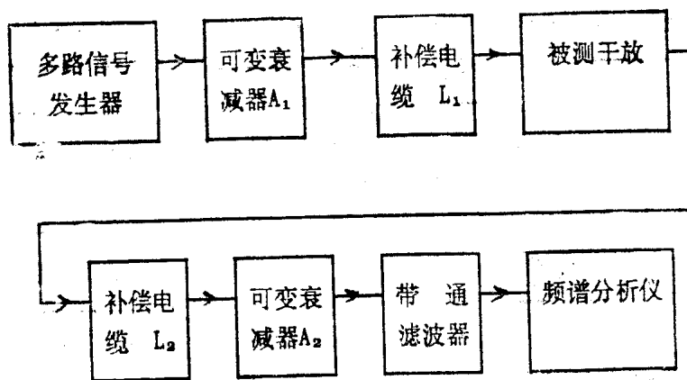
图9 C/CTB, C/CSO测量
