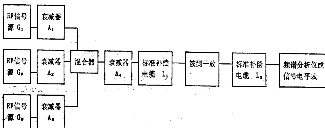
图3 AGC特性测量
