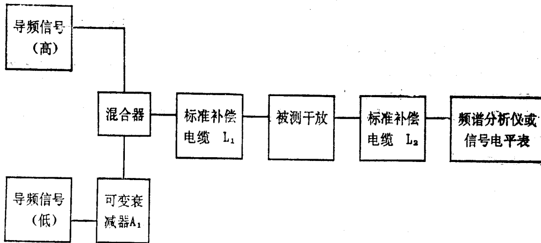
图4 ASC特性测量
