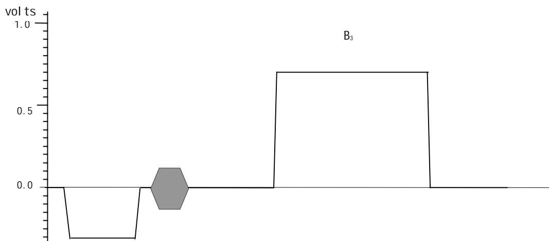
图 9 条脉冲 B_3 测试信号
