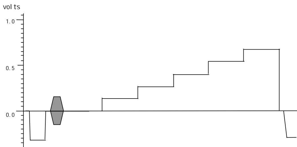
图 12 阶梯波信号
