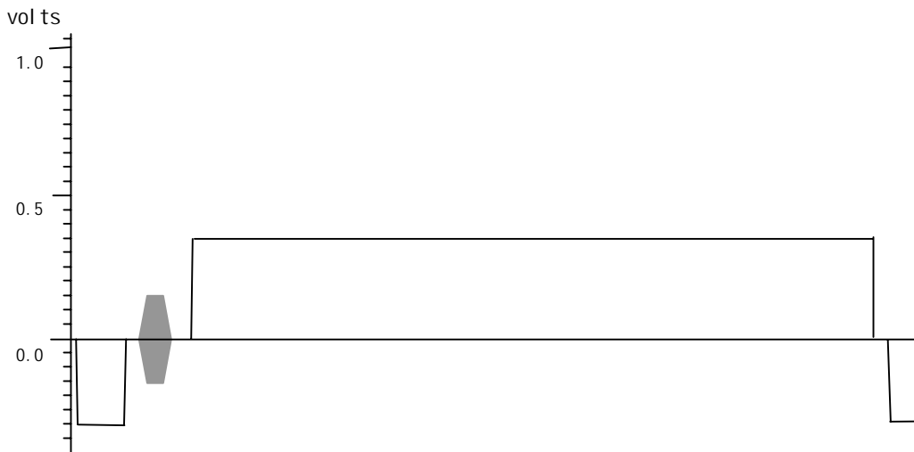
图 14 50%的平场信号
